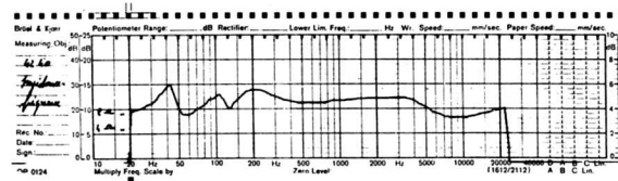
Courbe Impédance Fréquence
