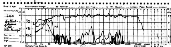
Réponse Amplitude - Fréquence et distorsion par Harmoniques 2 et 3
