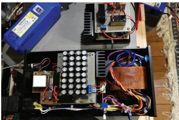
デジタルセパレーター用クロック Recording Equipment, Clock power.
